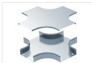
CRC / TCRC Cruce canales / Tapa cruce canales Conforme norma UNE-EN 61537
