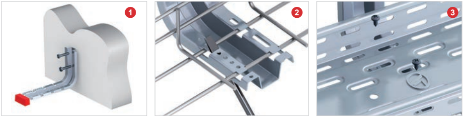
Ventajas del nuevo sistema de soportes omega multifunción
